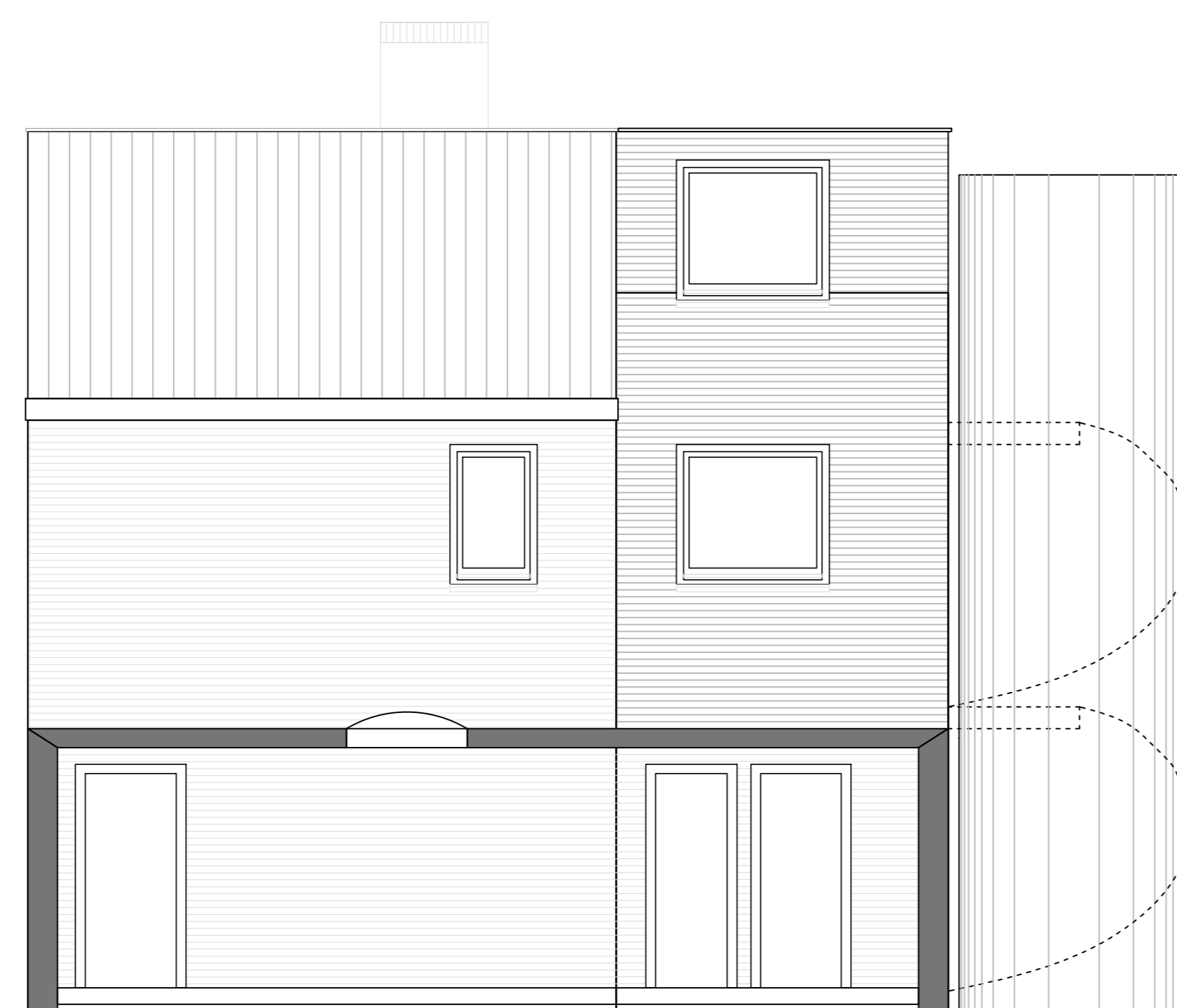
rechter-zijgevel
